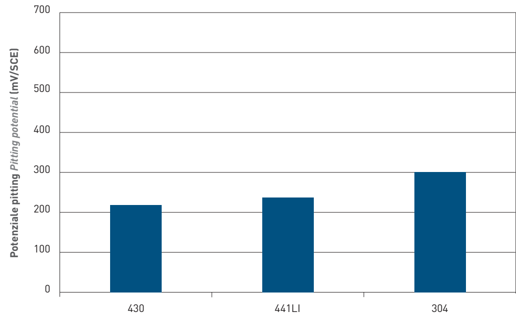
Valori indicativi del potenziale critico di pitting secondo standard ASTM G61 (NaCl 3.56%. T amb ). Typical values of critical pitting potential according to ASTM G61 standard (NaCl 3.56%, RT).
