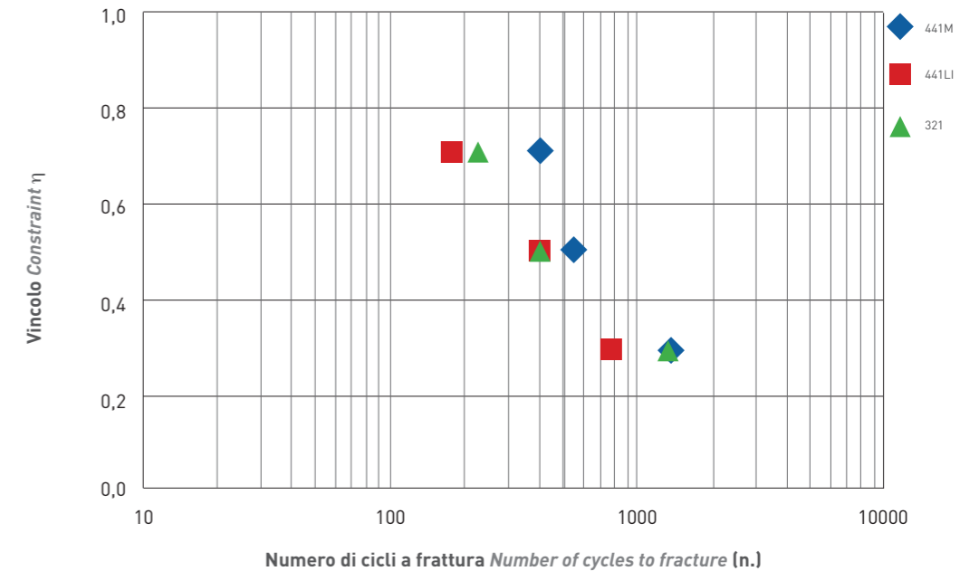
Diagramma di resistenza alla fatica termica ( \eta vincolo meccanico) - numero di cicli. Thermal fatigue resistance diagram ( \eta mechanical constraint) - number of cycles.
