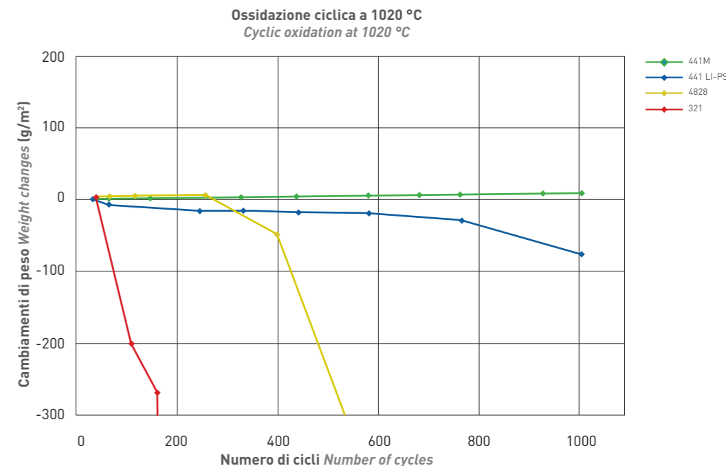
Variazione di peso per unità di superficie in funzione del numero di cicli termici cui è sottoposto il materiale (un ciclo: 25' alla temperatura di prova, 5' a temperatura ambiente). Weight change per unit area based on the number of thermal cycles to which the material is subjected (one cycle: 25' at test temperature, 5' at room temperature).
