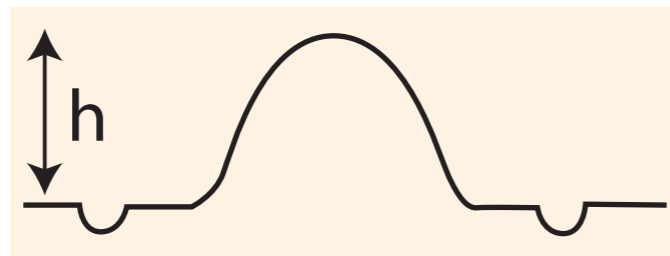
Schema del calcolo dell'indice Erichsen. Calculation method of Erichsen Index.
